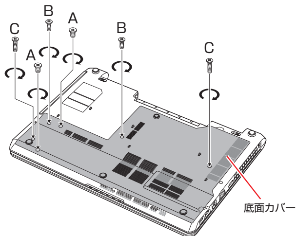
ネジ A (HDD 刻印用) ネジ B ネジ C
